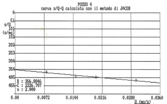
Figura 9 – Curva s/Q-Q calcolata con il metodo di Jacob
