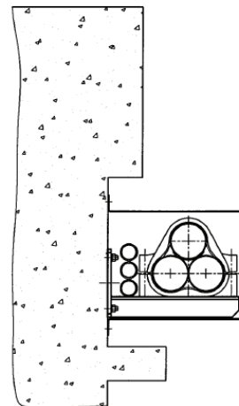
Staffaggio cavi A.T. sulla fiancata del ponte/viadotto
