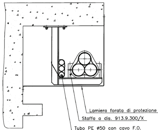
Staffaggio cavi A.T. sotto la soletta in cemento armato
