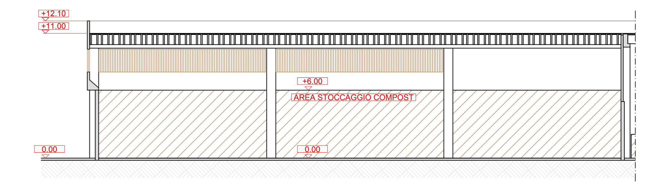
SEZIONE D-D
