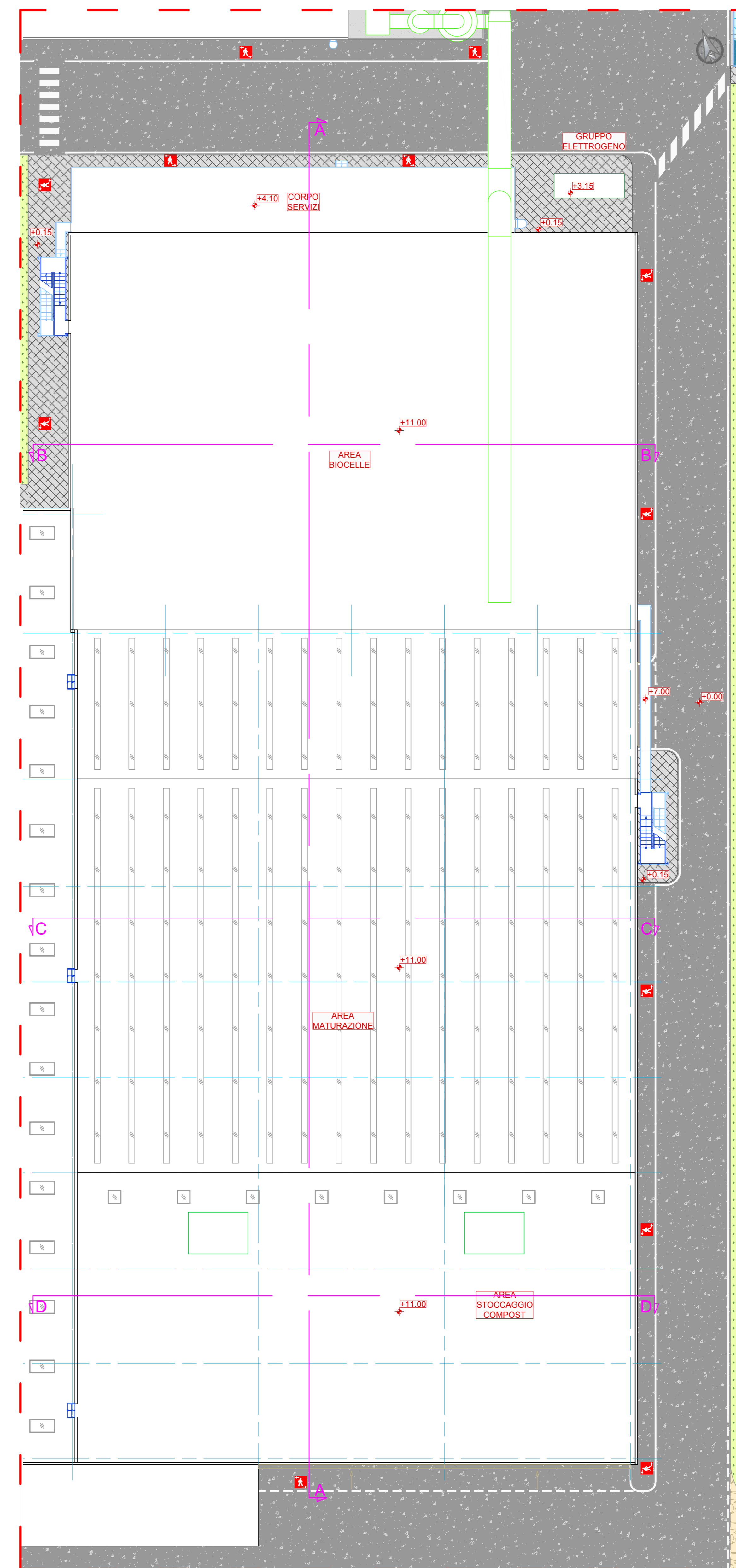
PIANTA COPERTURE
