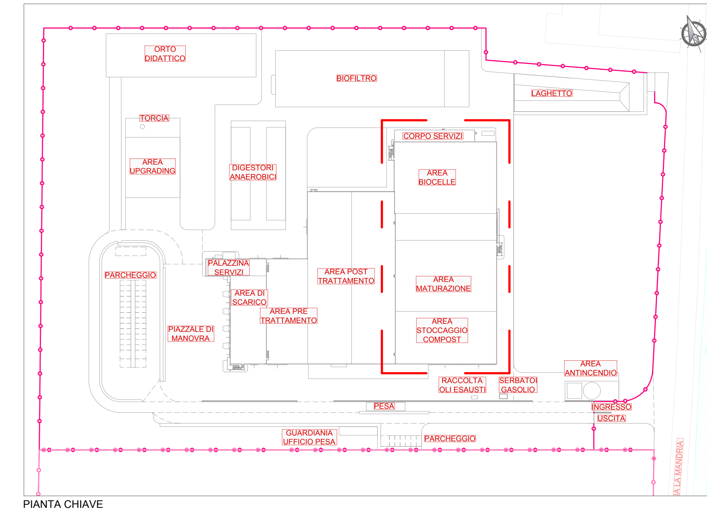
PIANTA CHIAVE
